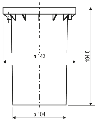
Einbautopf
