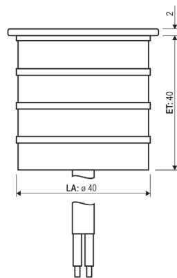
mit Einbautopf
