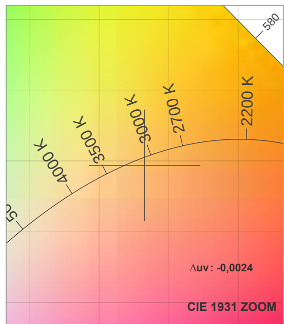
CRI: 86,6 (R1-R8)
