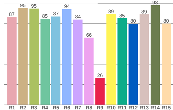
CRI: 86,6 (R1-R8)
