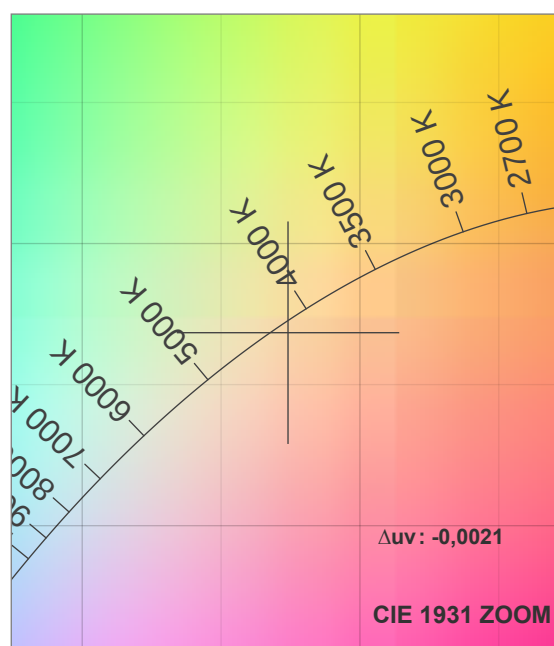
CRI: 83,8 (R1-R8)
