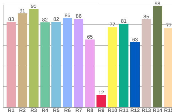
CRI: 83,8 (R1-R8)
