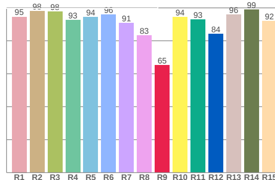
CRI: 93,4 (R1-R8)
