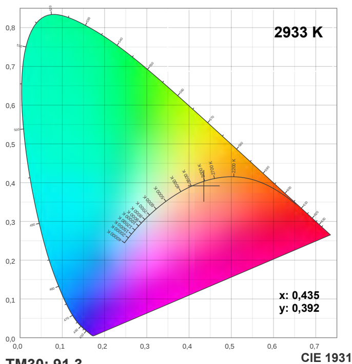
CRI: 93,4 (R1-R8)
