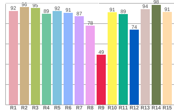
CRI: 90,2 (R1-R8)
