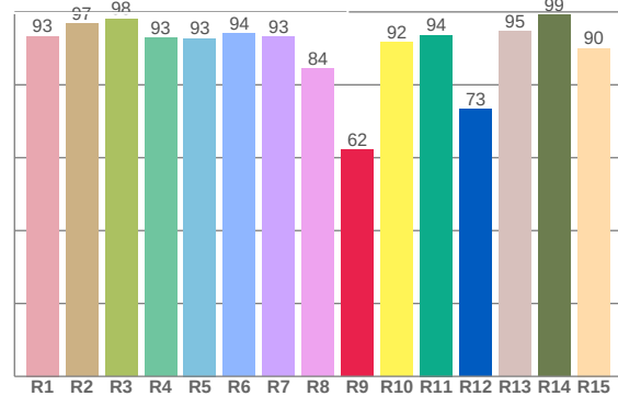
CRI: 93,2 (R1-R8)
