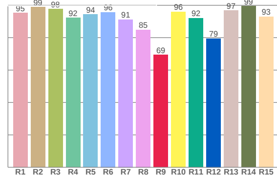
CRI: 93,8 (R1-R8)
