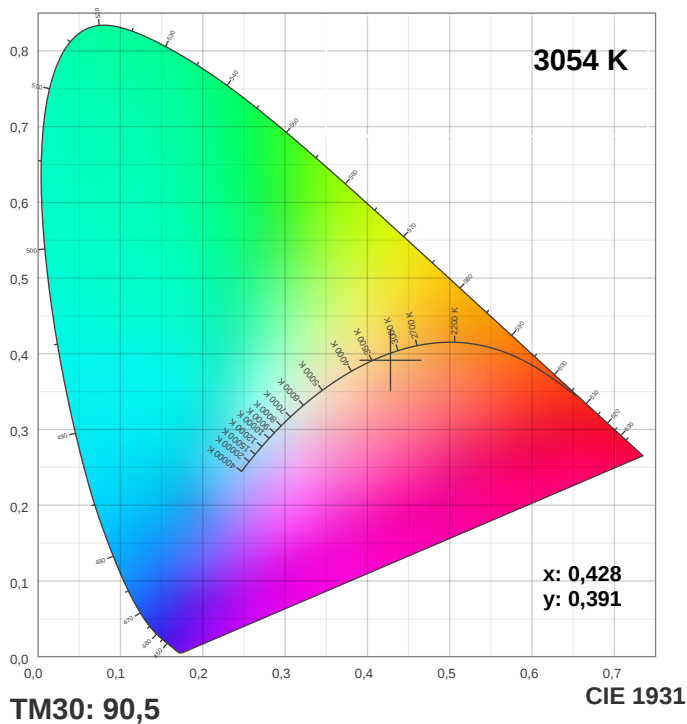
CRI: 93,8 (R1-R8)
