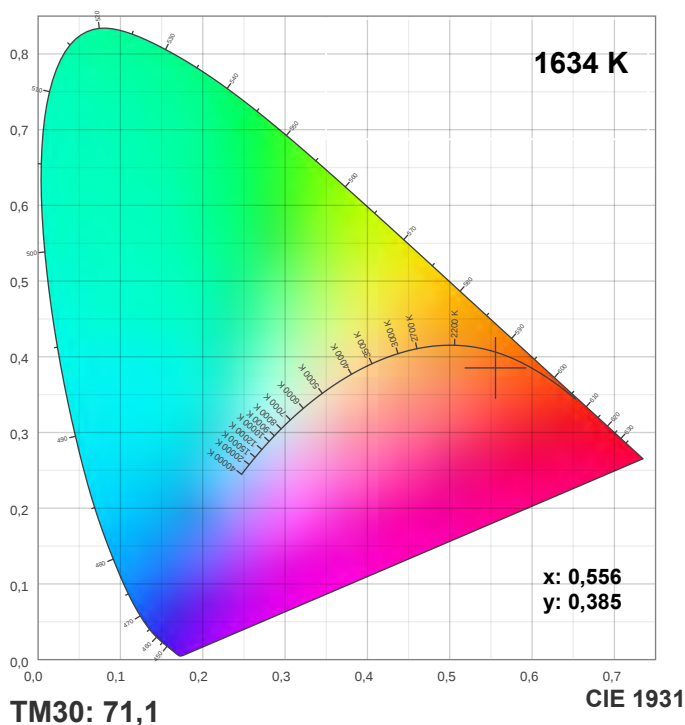
CRI: 84,2 (R1-R8)
