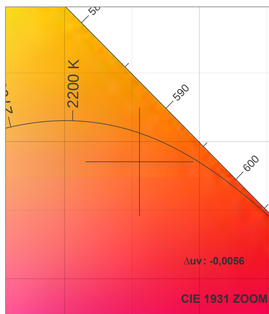
CRI: 84,2 (R1-R8)
