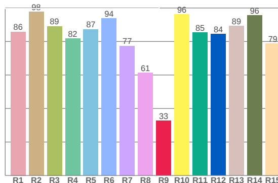
CRI: 84,2 (R1-R8)
