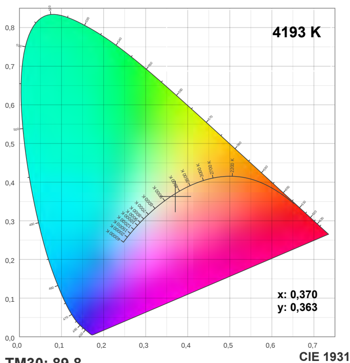
CRI: 94,3 (R1-R8)
