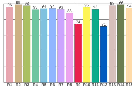
CRI: 94,3 (R1-R8)
