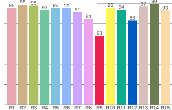
CRI: 93,9 (R1-R8)
