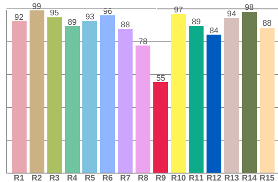
CRI: 91,1 (R1-R8)
