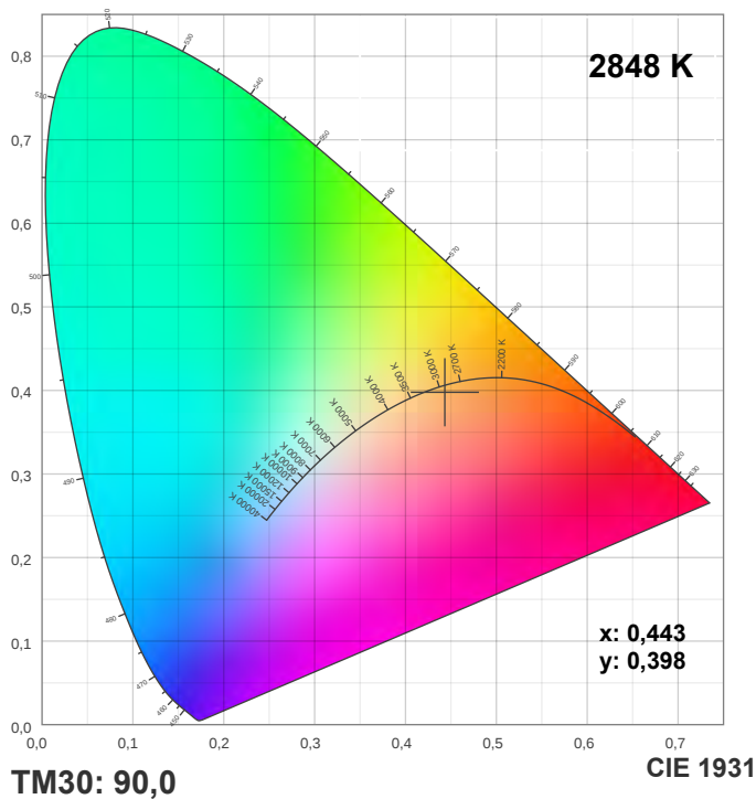
CRI: 91,1 (R1-R8)
