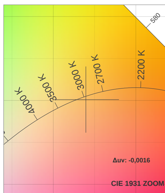
CRI: 93,8 (R1-R8)
