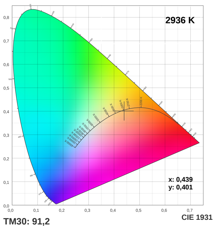
CRI: 93,8 (R1-R8)
