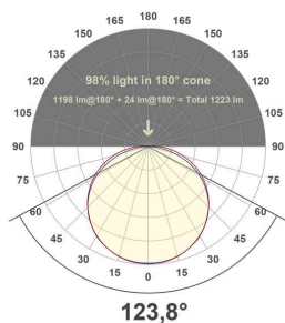
SK542460280125_PD
