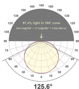
SK542460280125_PD-6500K
