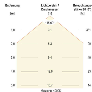
LDQ170125_KD-4000K
