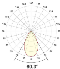
HSB6520040_PD-HBR80100
