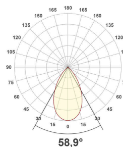
ED54504925_PD-5700K
