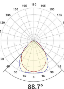
APSU620125_PD-33W-mix
