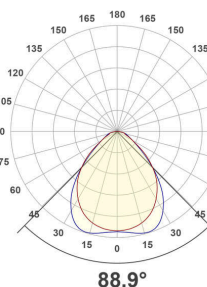
APSU620125_PD-33W-3000K
